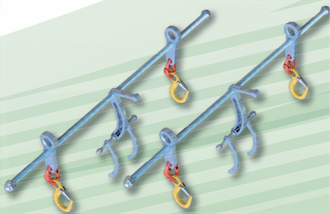
■ 標準タイプセット(ハングバー2本+間隔治具2組)
