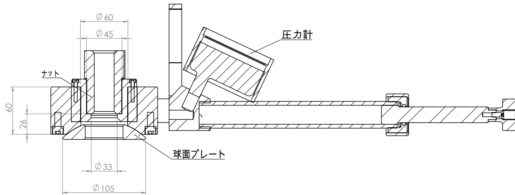
断面図 A-A
