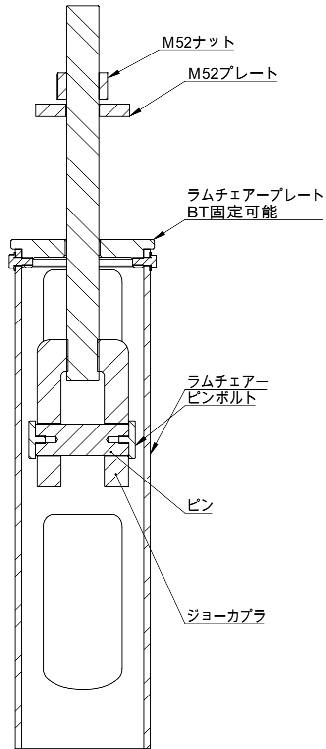
断面図 C-C
