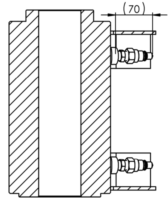
断面図 A-A
