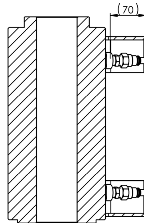
断面図 A-A
