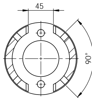
断面図 C-C
