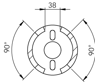
断面図 A-A
