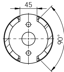
断面図 F-F スケール 1 : 4
