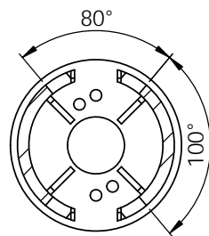
断面図 H-H
