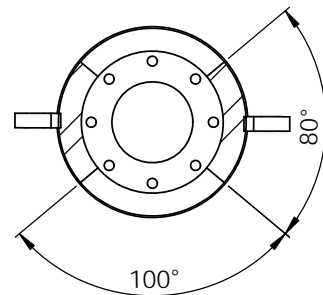
断面図 A-A スケール 1 : 7
