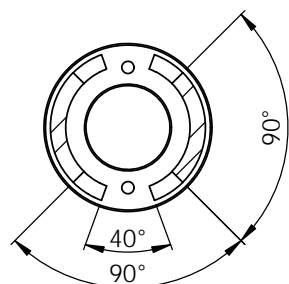
断面図 B-B スケール 1 : 7
