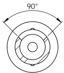
断面図 A-A
