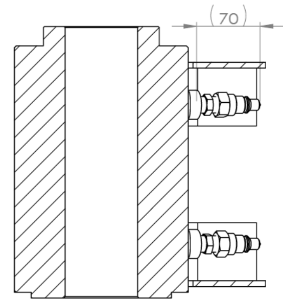
断面図 A-A
