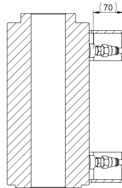
断面図 A-A
