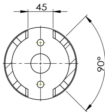
断面図 F-F スケール 1 : 4
