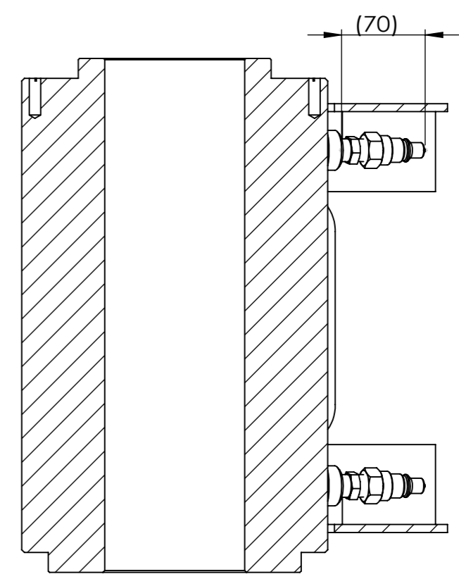
断面図 A-A
