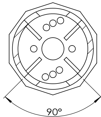
断面図 E-E スケール 1:4
