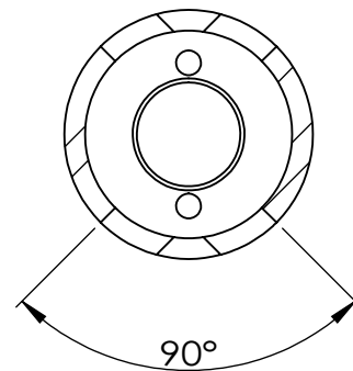
断面図 A-A スケール 1 : 4
