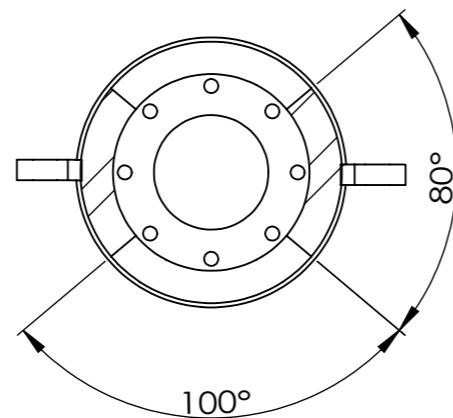
断面図 A-A スケール 1 : 7
